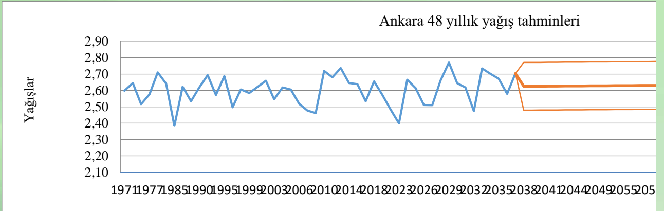
Grafik 3.4. Ankara 2019-2066 yıllarına ait yıllık yağış tahminleri
