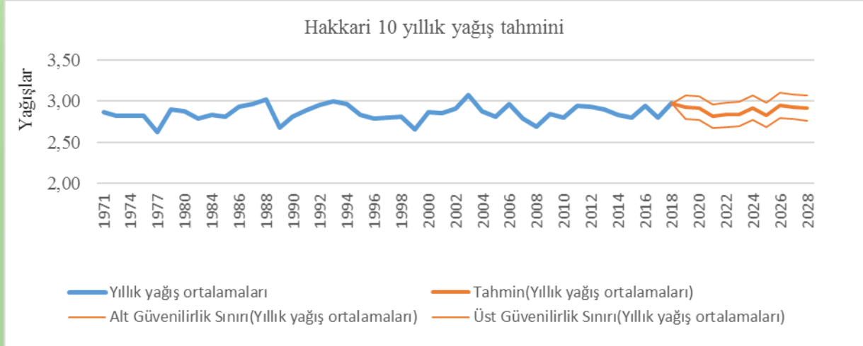
Grafik 3.13. Hakkâri 2019-2028 yıllarına ait yıllık yağış tahminleri
