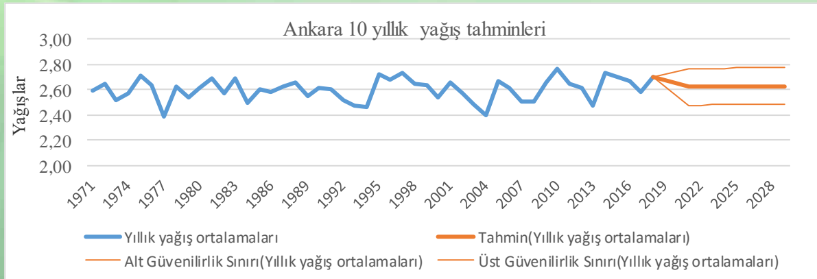
Grafik 3.1. Ankara 2019-2028 yıllarına ait yıllık yağış tahminleri
