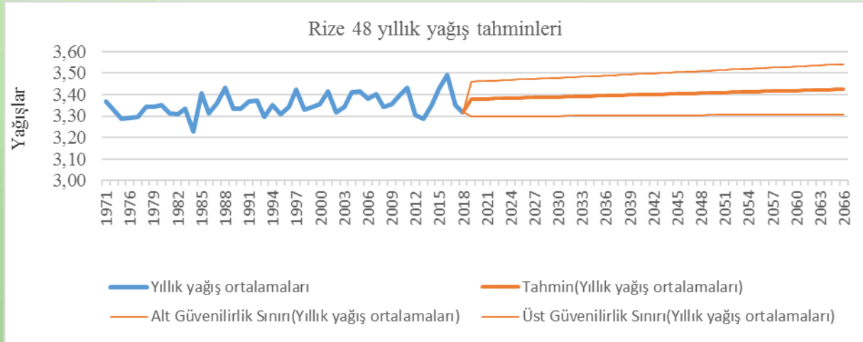
Grafik 3.8. Rize 2019-2066 yıllarına ait yıllık yağış tahminleri
