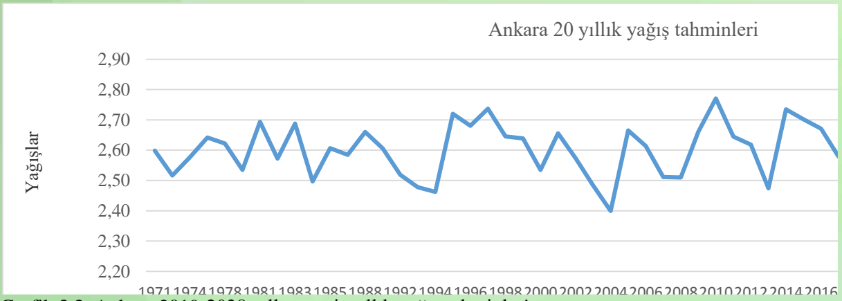
Grafik 3.3. Ankara 2019-2038 yıllarına ait yıllık yağış tahminleri
