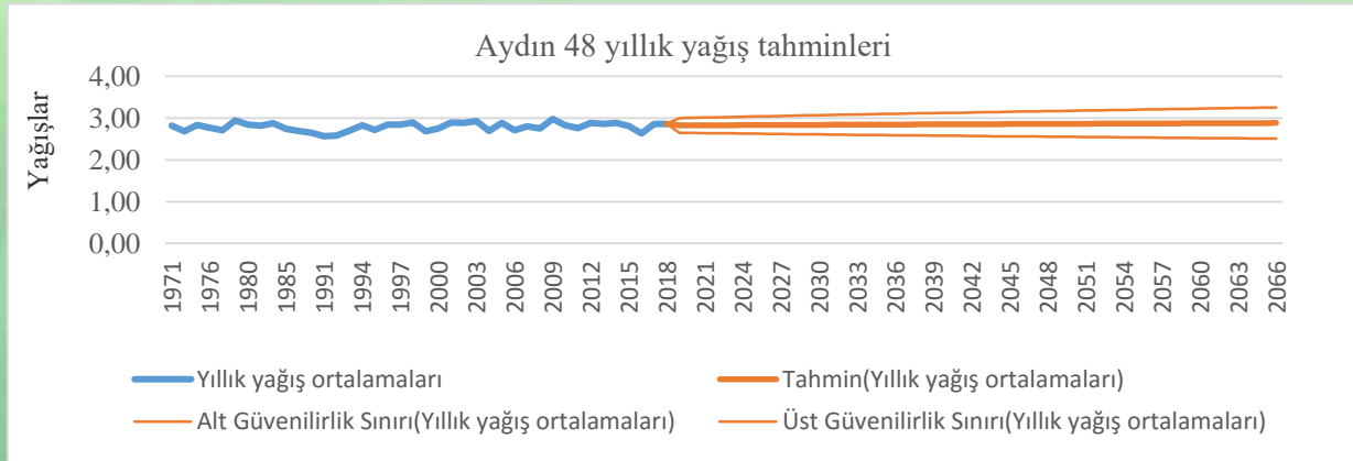
Grafik 3.12. Aydın 2019-2066 yıllarına ait yıllık yağış tahminleri
